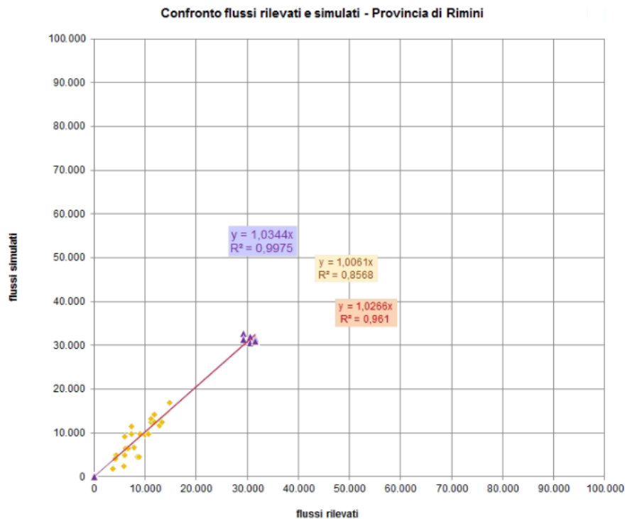
Figura 11: Risultati della calibrazione: correlazione tra flussi rilevati e simulati – rete provinciale (Elaborazione META srl)
