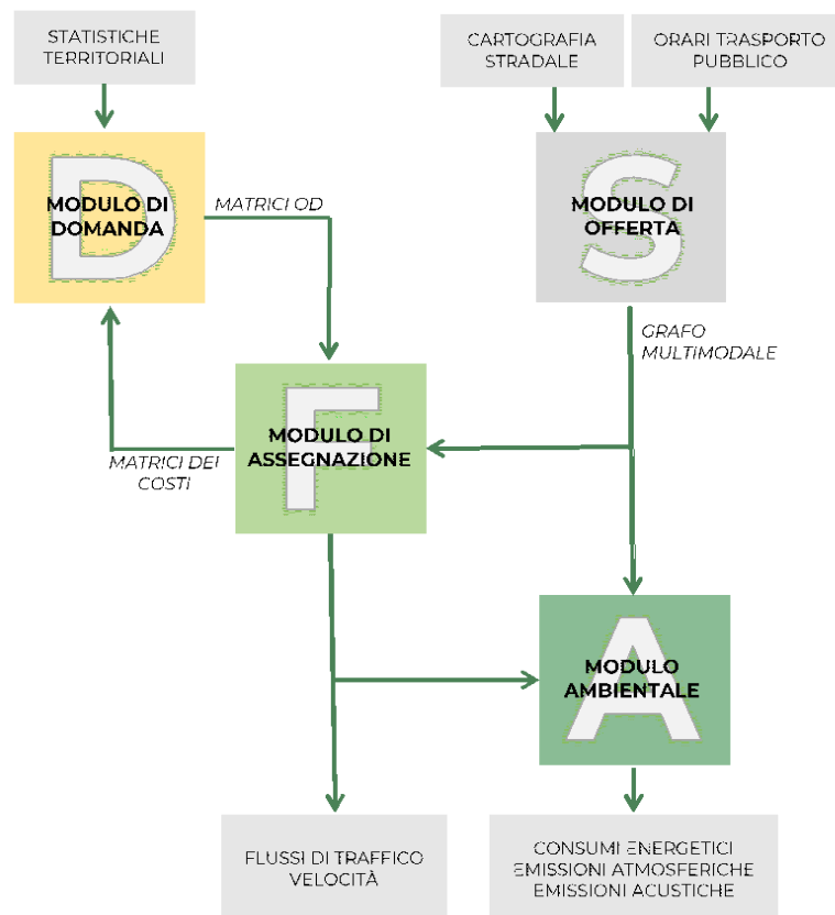
Figura 7: Schema logico del modello di simulazione di traffico (Elaborazione META srl)
