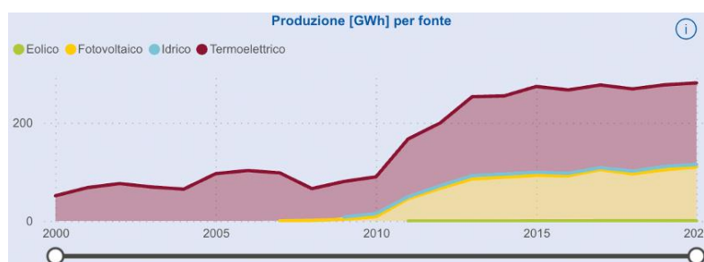
All. 7 Figura 14: Produzione di energia elettrica per tipologia di fonte- Totale 281,2 Wh 29
