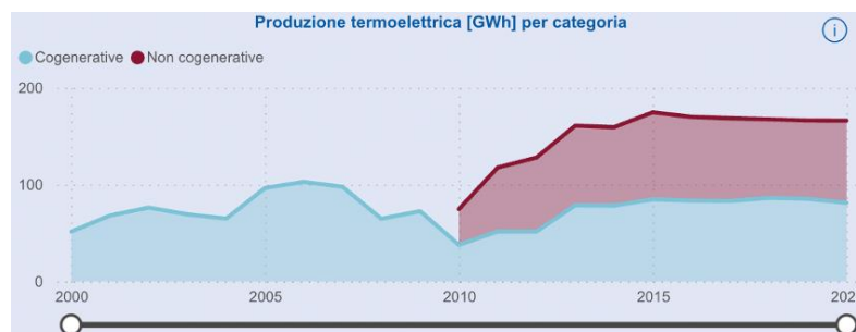
All. 7 Figura 15: Produzione di energia termoelettrica per tipologia di fonte- Totale 166,0 GWh 30
