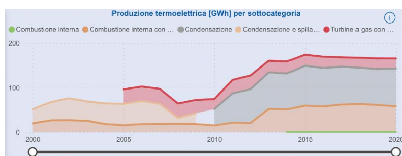
All. 7 Figura 16: Produzione termoelettrica per sottocategoria in provincia di Rimini 31
