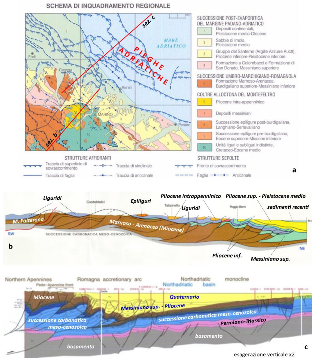
ALL. 4 Figura 2: a) Schema geologico di sintesi dell’area d’interesse (da Carta Geologica d’Italia 1:50.000, Foglio 256 “Rimini”), con tracce delle sezioni b e c; b) Sezione geologica dal crinale tosco-romagnolo a Santarcangelo di Romagna (da Cerrina Feroni et al., 2002); c) sezione geologica dall’Appennino Romagnolo al Mar Adriatico (da Fantoni e Franciosi, 2010)
