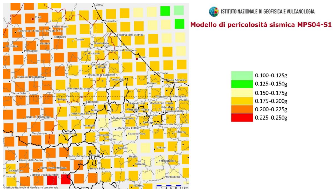
All. 4 Figura 13: mappa di pericolosità sismica di base per la Provincia di Rimini e aree limitrofe, TR= 475 anni (Gruppo di lavoro MPS, 2004); i colori indicano le classi di a_g , accelerazione di picco su suolo rigido e pianeggiante, espressa in percentuale dell'accelerazione di gravità g
