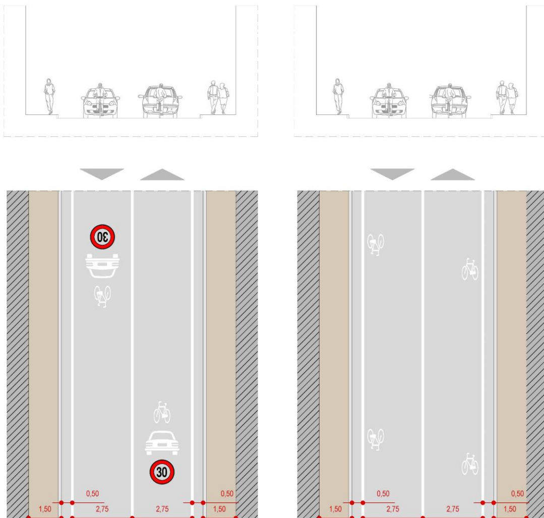
Figura 3.2: Schemi tipologici di strade promiscue
