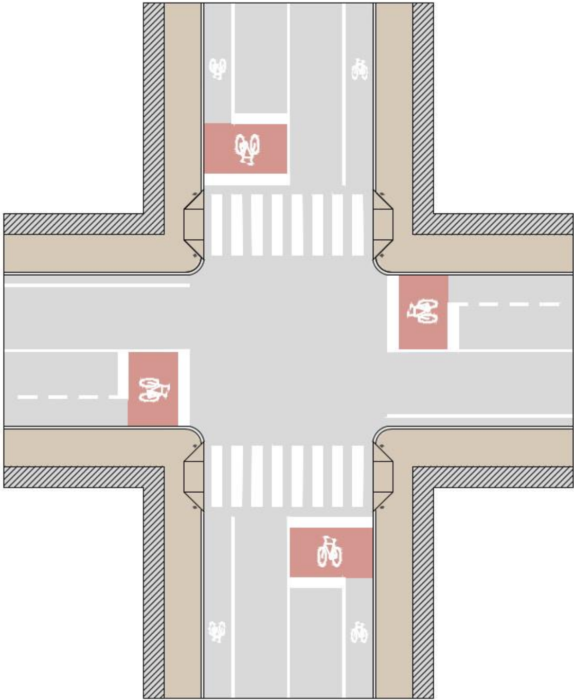
Figura 3.5: Schema tipologico di corsie ciclabili in prossimità di intersezione.
