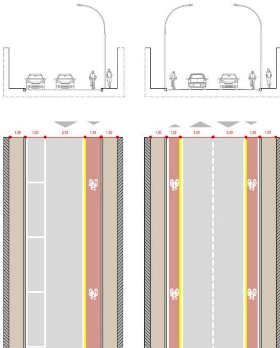
Figura 3.3: Schemi tipologici di strade con corsie ciclabili
