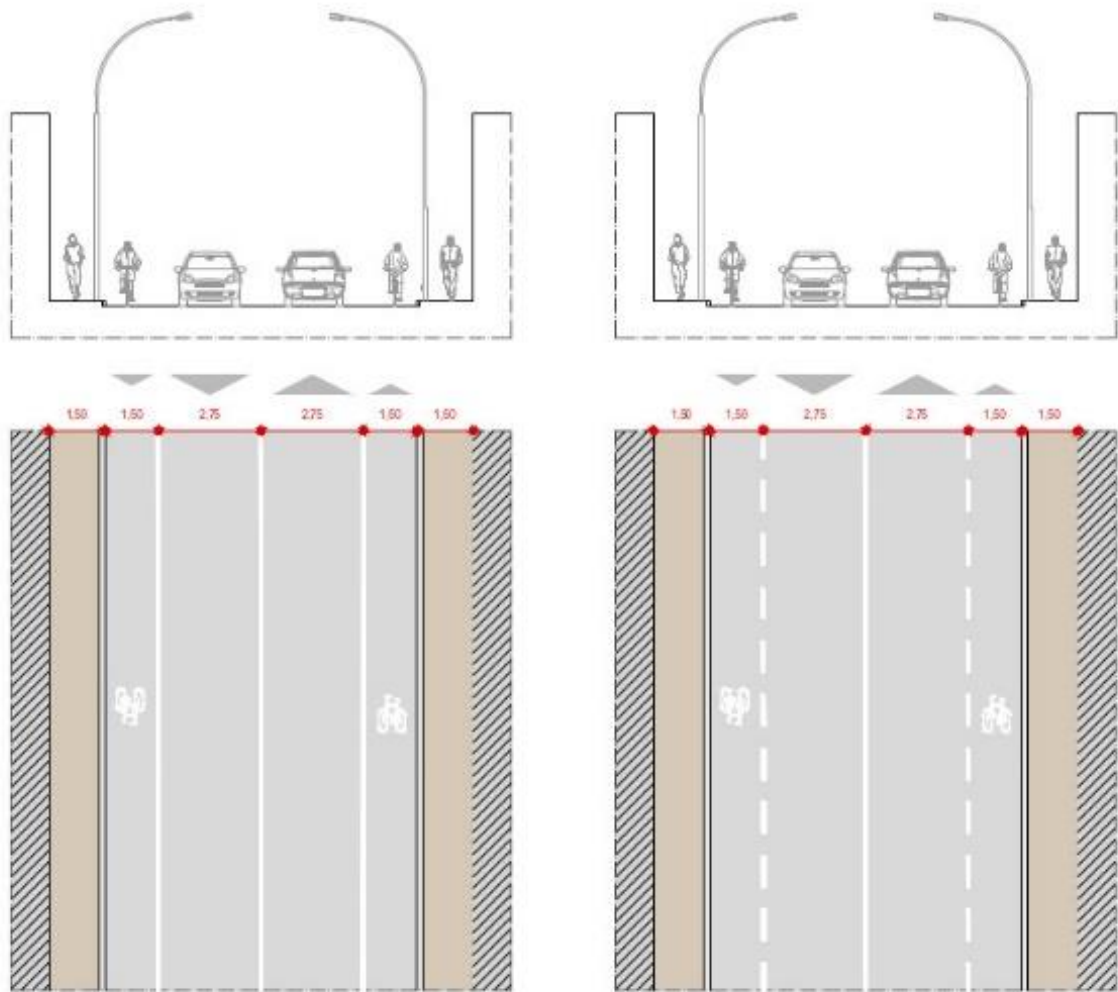
Figura 4.3: Schemi tipologici di strade con corsie ciclabili
