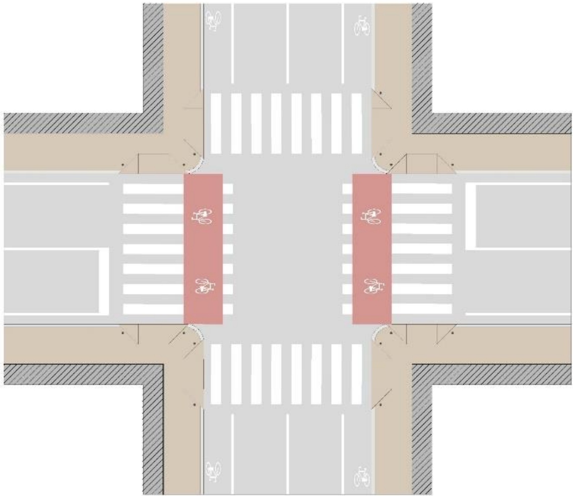
Figura 3.5: Schema tipologico di attraversamenti ciclopeditoni in prossimità di intersezione
